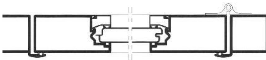
Sección puerta abisagrada 1 hojal
