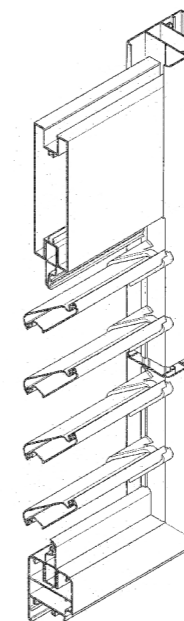
Lama Móvil
